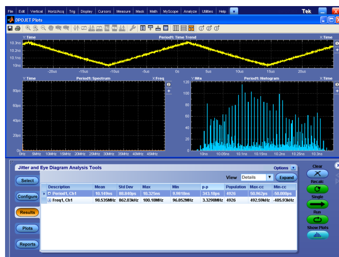
Расширенные измерения джиттера, глазковых диаграмм и временных характеристик.
